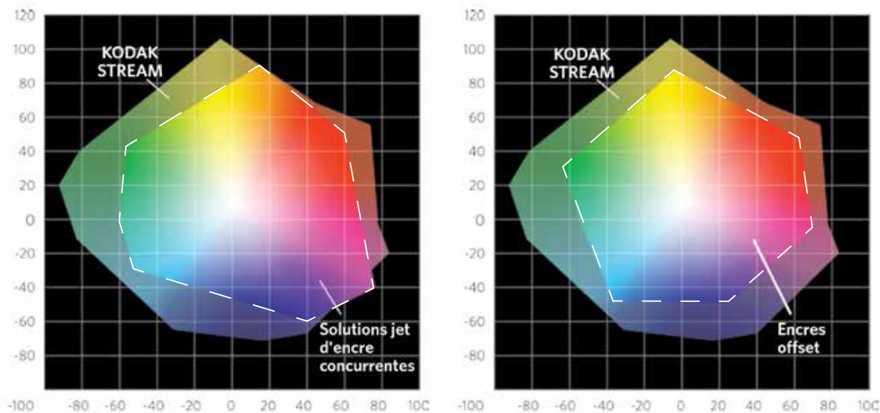
Figure 4 - Comparaison de la gamme chromatique par rapport à l'offset : la gamme chromatique des encres Kodak est bien plus large que celle des encres offset
